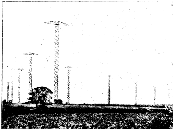
STAZIONE RICEVENTE A FASCIO DI BRIDGWATER COSTRUITA DALLA MARCONI'S WIRELESS TELEGRAPH COMPANY LTD. PER L'UFFICIO GENERALE POSTE INGLESIS SU SISTEMA MARCONI ONDE CORTE.
